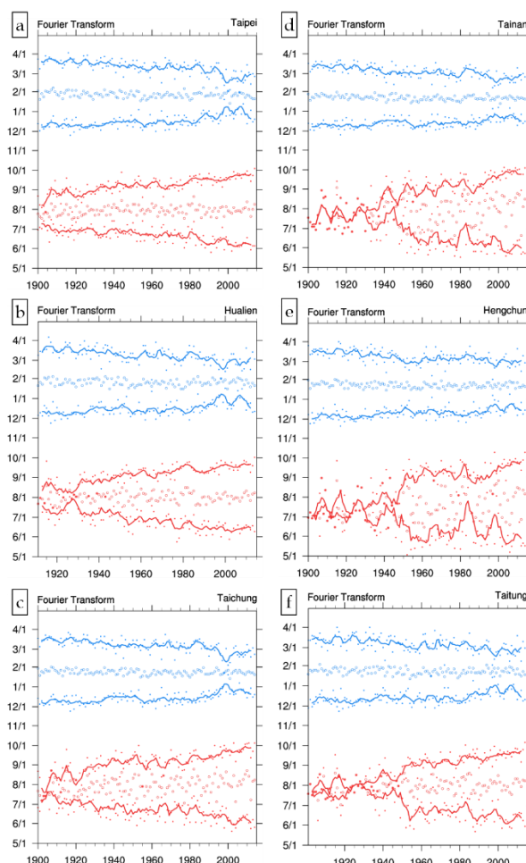
圖2 以Fourier Transform方法計算台灣六個百年測站所定義出的夏季(紅色圓點)、冬季(藍色圓點)之始末日期。線為五年移動平均的結果。圓環為峰值日期。橫軸為年份，縱軸為日期。
