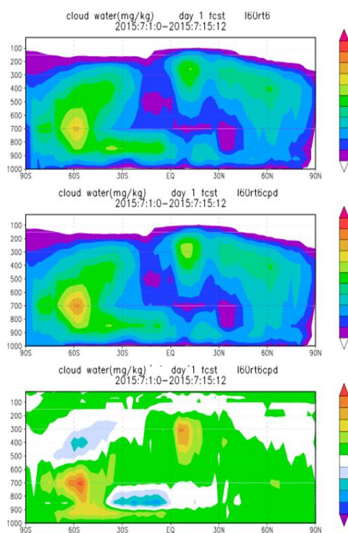
圖 3 2015/7/1-15 期間的雲水 24hr 預報平均場作業版(b)為測試版(c)為測試版-作業版的差值(y-z 垂直剖面。單位為 mg/kg)。
