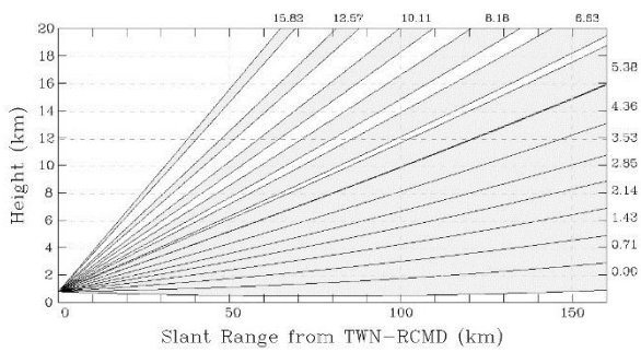
圖3 RCMD 雷達較佳掃描策略之13個觀測仰角。
