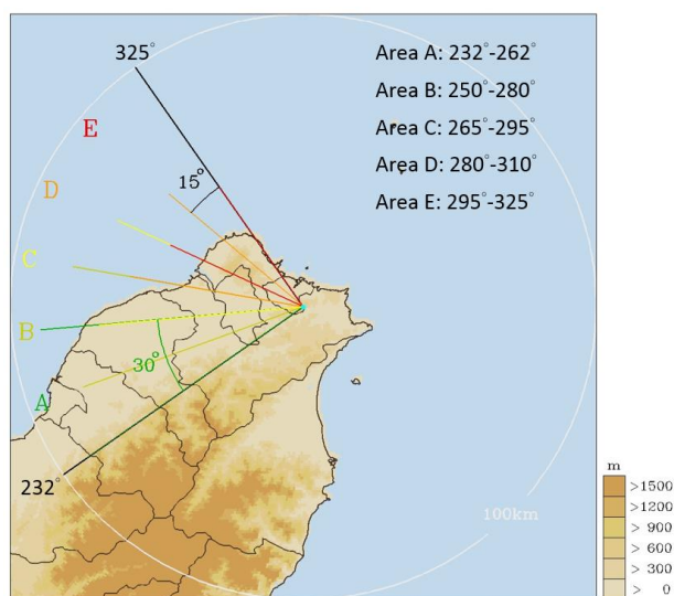
圖6 RCMD雷達針對觀測夏季午後對流系統進行 RHI 掃描之 A-E 等五個區域，各區域觀測方位角範圍如圖右上角所示。
