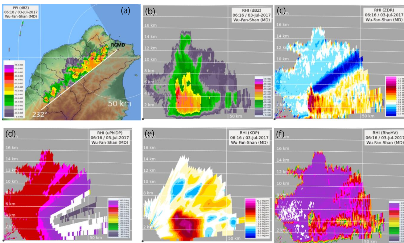
圖7 2017年7月3日 C波段RCMD雷達進行對流胞體積掃描之(a)06:17 UTC 2.4° PPI 觀測回波圖；(b)為 06:17 UTC 方位角 232° RHI 掃描觀測回波；(c)-(f)同圖(a)，但為(c)差異反射率、(d)差異相位差、(e)比差異相位差和(f)相關係數。雷達位於圖中黑點位置。
