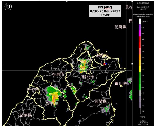
圖5 2017年7月10日(a) 07:06 UTC C波段RCMD雷達與(b) 07:05 UTC S波段RCWF雷達之 0.5^{\circ} PPI 觀測回波圖。
