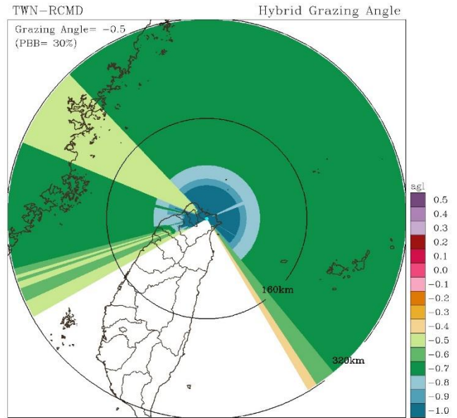
圖2 RCMD 雷達於觀測仰角 -1.0^{\circ} – 0.5^{\circ} 間之波束於標準大氣下之可觀測仰角整合圖粗線。顏色表示該位置之最低可用仰角。
