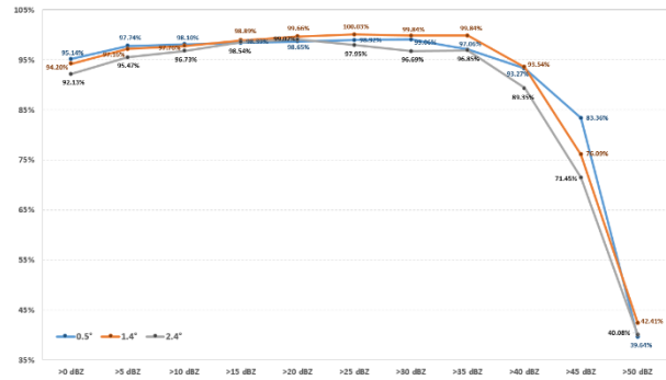
圖4 RCMD雷達於 2017年6月1日至4日期間，仰角 0.5^{\circ} 、 1.4^{\circ} 、 2.4^{\circ} 之都卜勒掃描模式相對於監測掃描模式之觀測資料比例。
